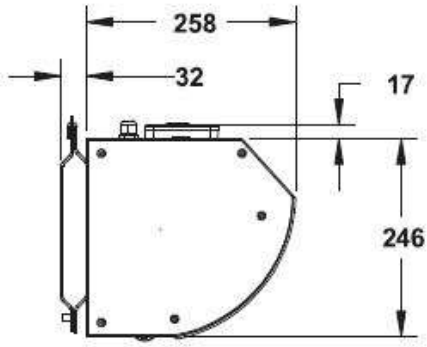
DEKORATİF TİP LED SERİ ELEKTRİK İSİTİCİLİ HAVA PERDELEİ EBAT VE AĞIRLIK TABLOSU
