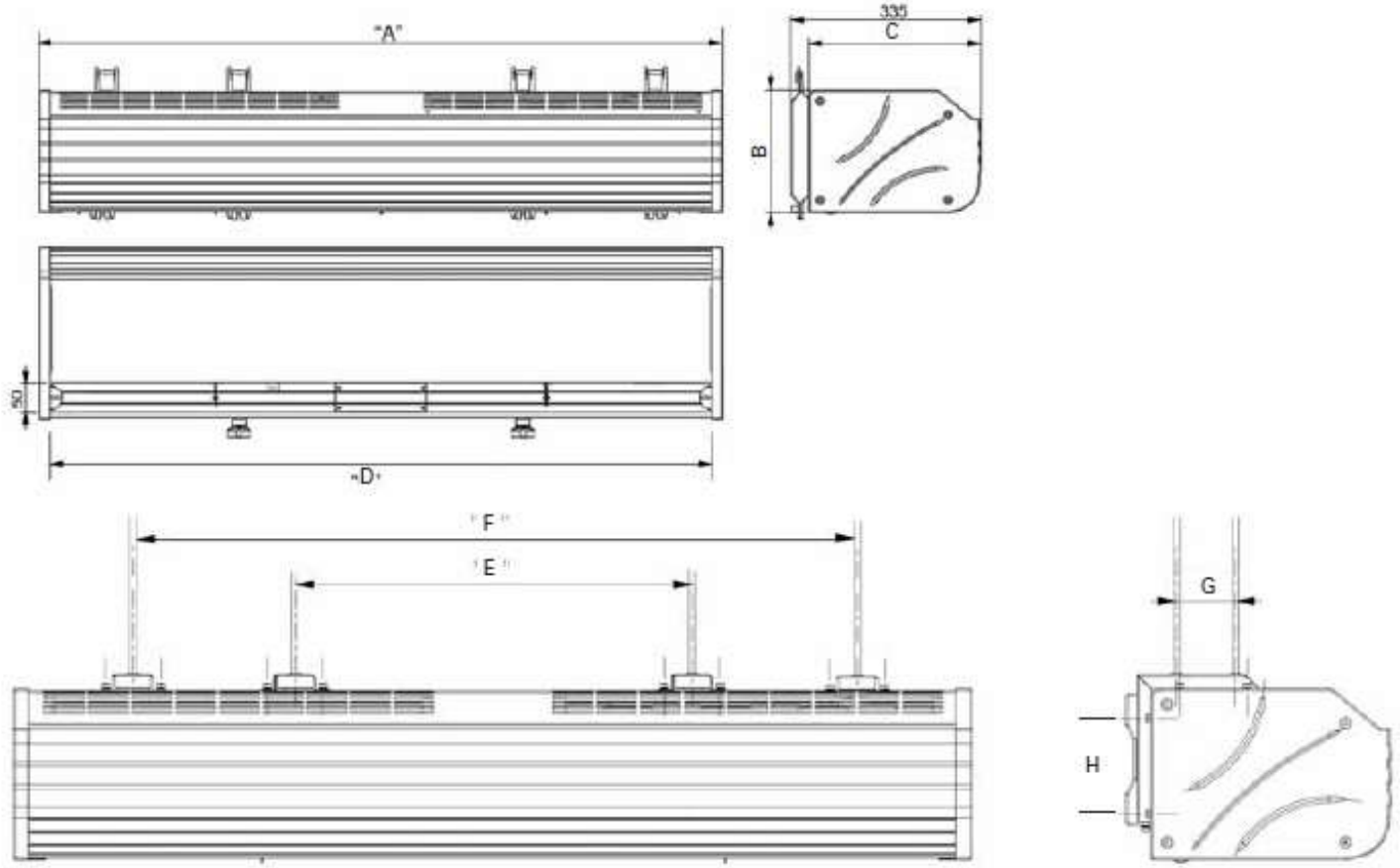
GENEL TİP ELEKTRİKLİ ISITICILI HAVA PERDELERİ EBAT VE AĞIRLIK TABLOSU
