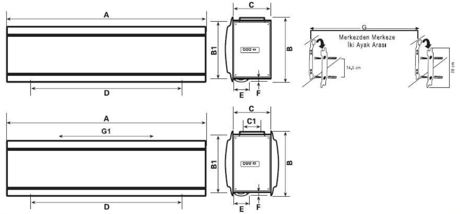
ECO ELEKTRİKLİ ISITICILI HAVA PERDELERİ EBAT VE AĞIRLIK TABLOSU
