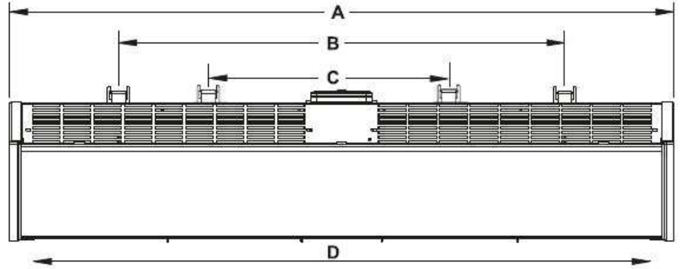
DEKORATİF TİP LED SERİ ELEKTRİKLİ ISITICILI HAVA PERDELEİ EBAT VE AĞIRLIK TABLOSU
